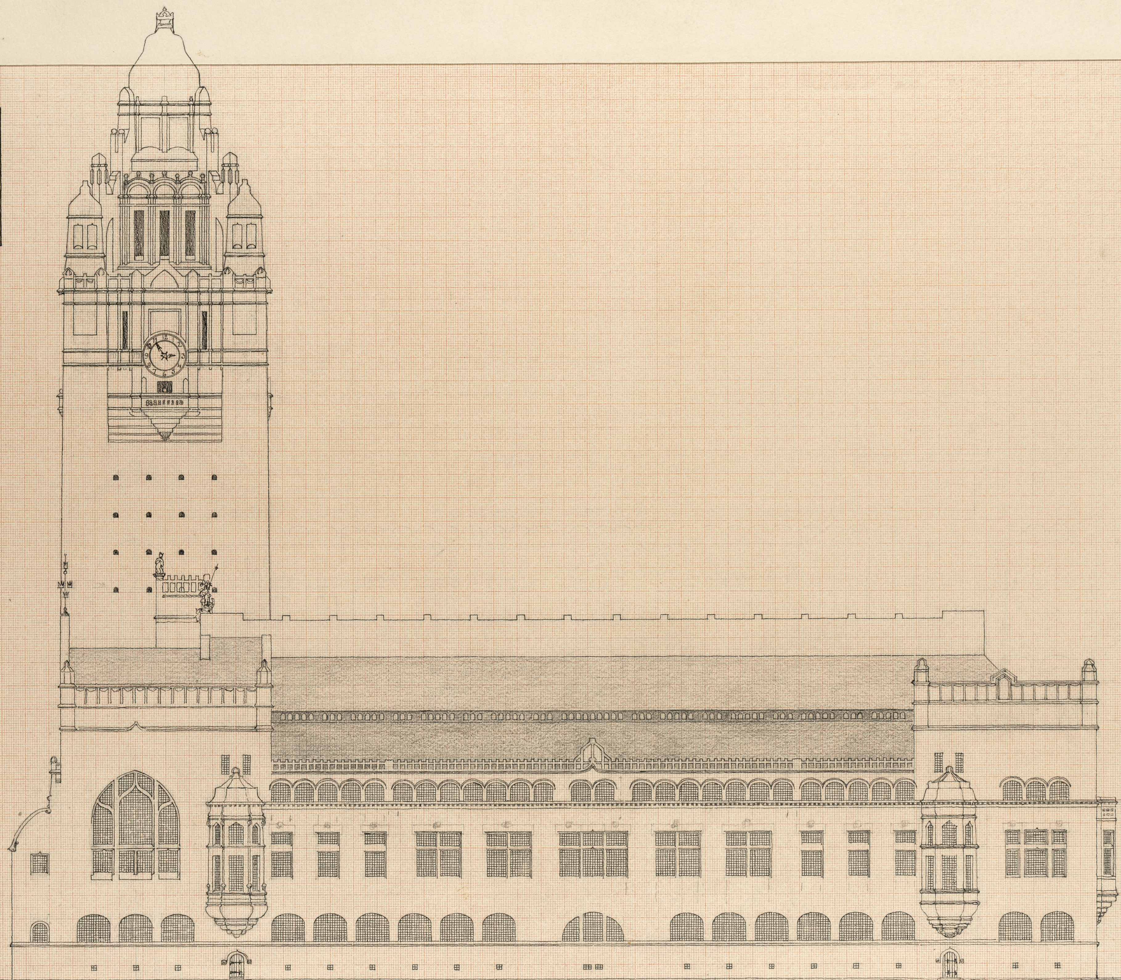
•MALÄRDROTTS RÅDHUSRITNING• •FASAD MOT HANDVERKAREGATAN• •PL. 18•
