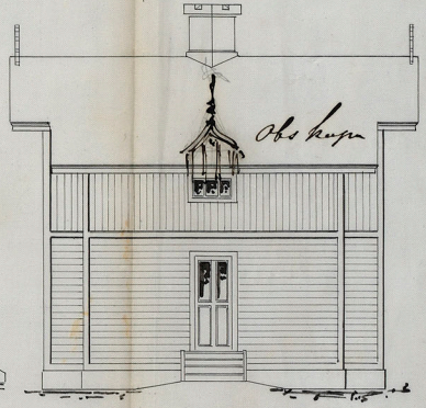
Sidofasad.
