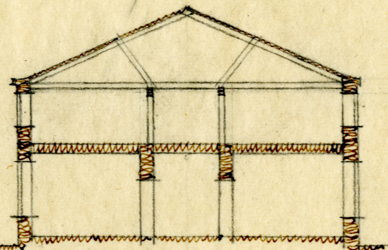
Sektion G-F.
