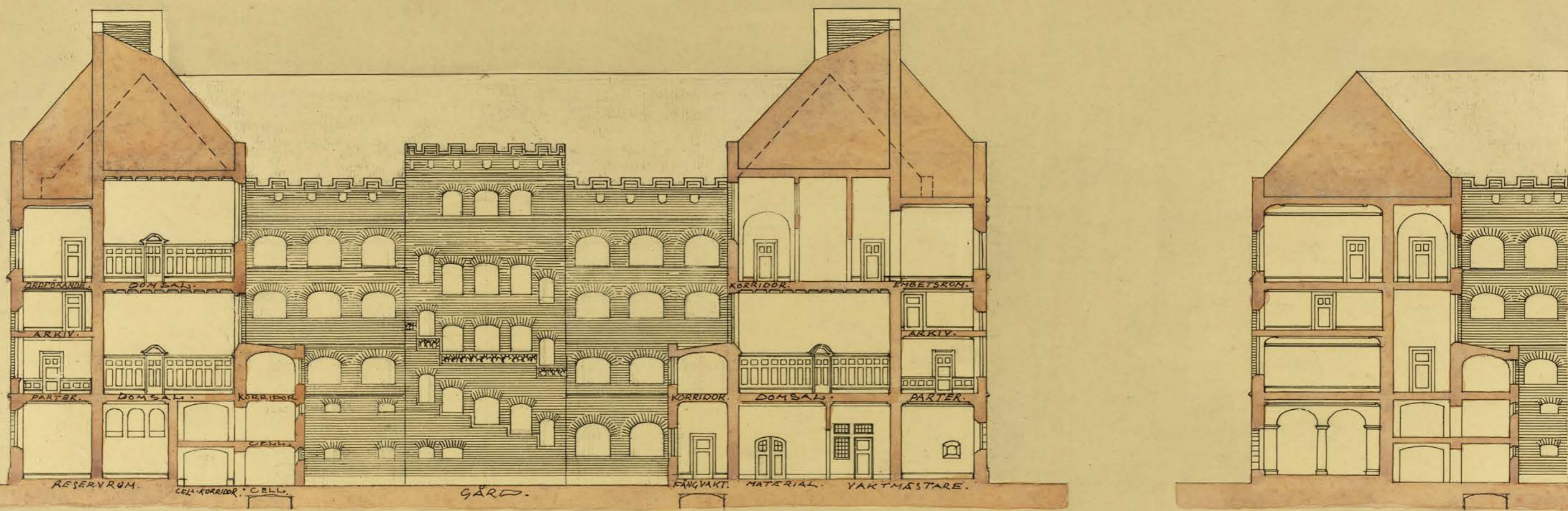
• TVÄRSEKTION • C-D •
