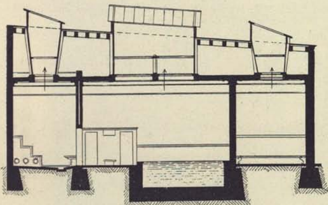
197. Folkskolebad på Östermalm, genomskärning.
