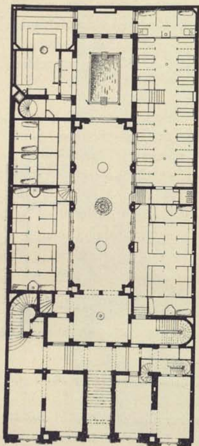
194. Sturebadet, plan af bottenvåningen.
