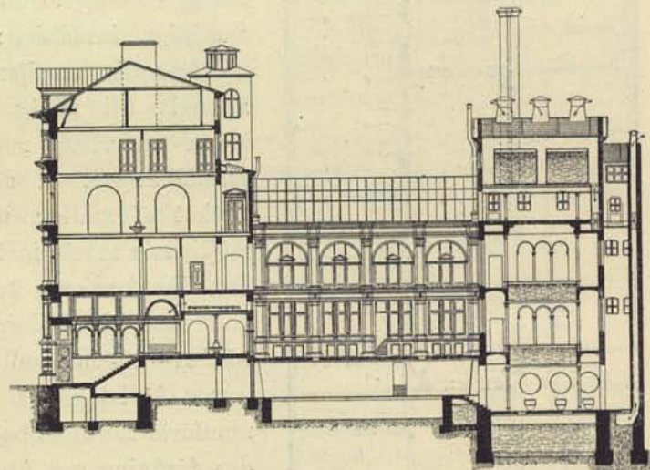
198. Sturebadet, längdgenomskäring af byggnaden.
