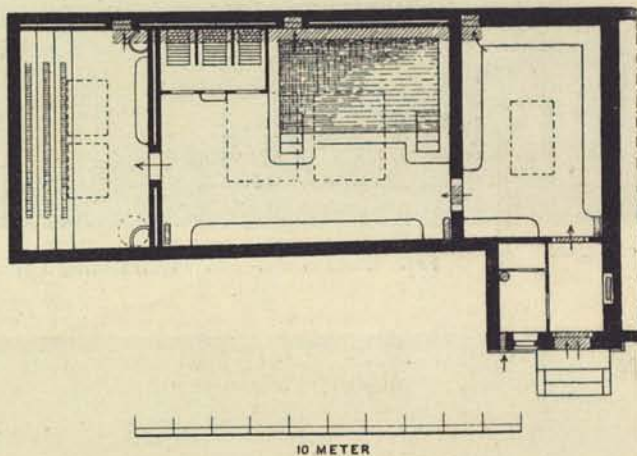
198. Folkskolebad på Östermalm, planritning.
