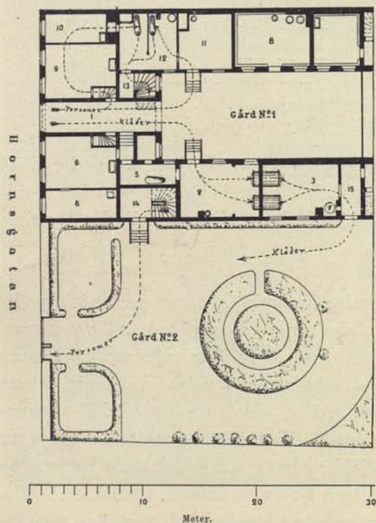
187. Plan af stadens desinfektionsanstalt.
