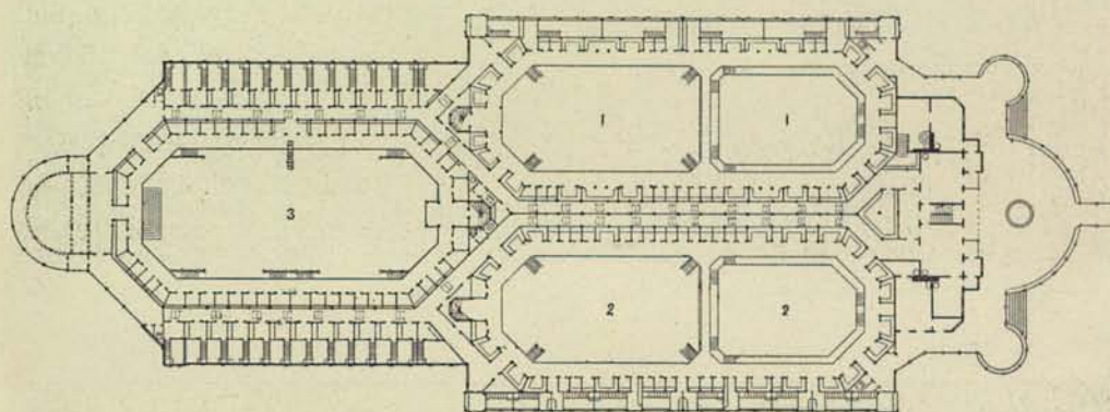
201. Stadens sim- och badinrättning i Norrström, plan.
