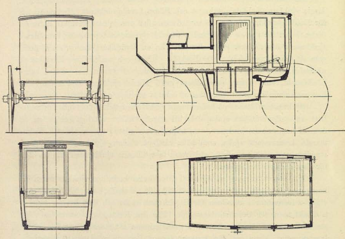
189. Sjuktransportvagn med rörlig sjukbår.
