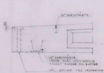
DETALJ A15B 1:10
