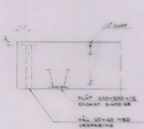
DETALJ C15B 1:10
