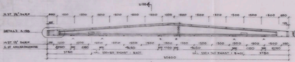
BALK 402 GB, 407 GB 1+1 ST 1:50
