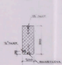
DETALJ D15B 1:10
