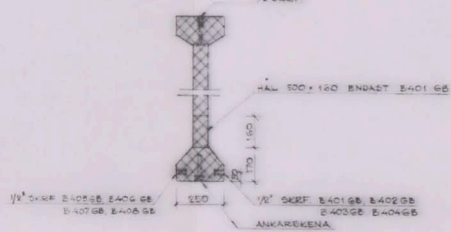
DETALJ C15B 1:10
