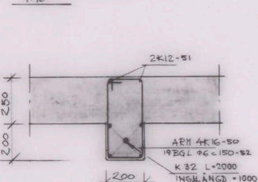
PELARE 508 G 1:10
