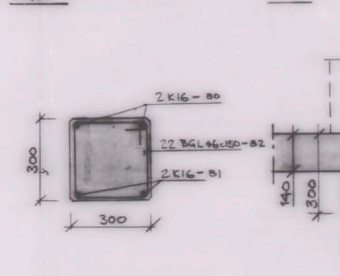
PELARE 404 G 1:10
