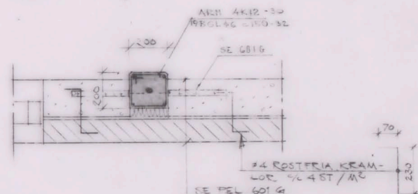
PELARE 505 G 1:10
