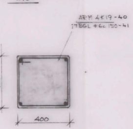
PELARE 507 G 1:10
