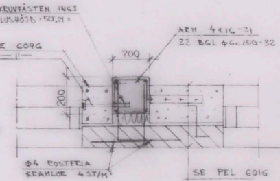
PELARE 515 G 1:10
