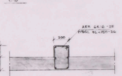
PELARE 506 G 1:10
