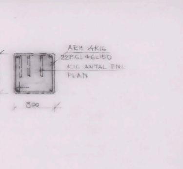
PELARE 614 G 1:10
