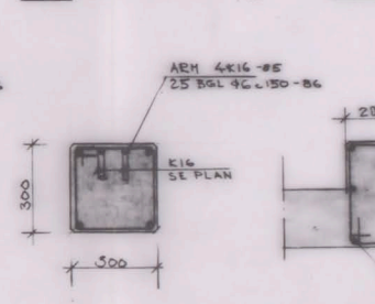
PELARE 406 G 1:10
