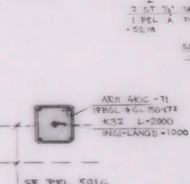
PELARE 512 G 1:10
