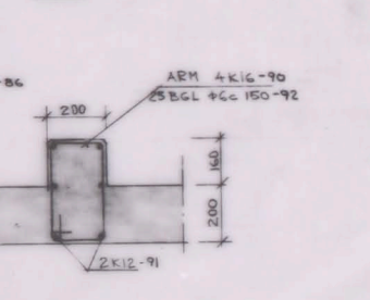
PELARE 407 G 1:10
