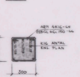
PELARE 511 G 1:10
