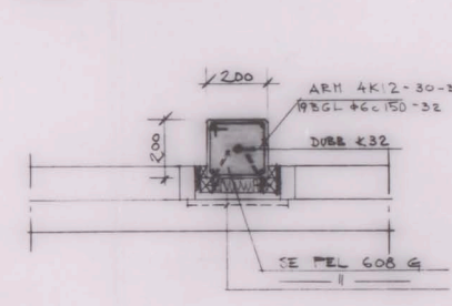
PELARE 503 G 1:10
