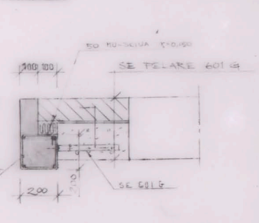
PELARE 606 G 1:10
