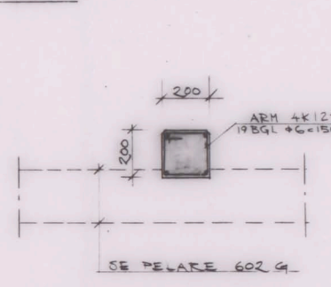
PELARE 603 G 1:10
