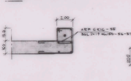
PELARE 509 G 1:10
