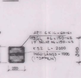
PELARE 510 G 1:10
