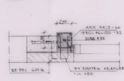
PELARE 502 G 1:10
