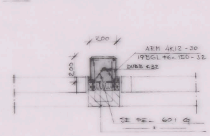
PELARE 501 G 1:10
