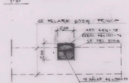
PELARE 401 G 1:10
