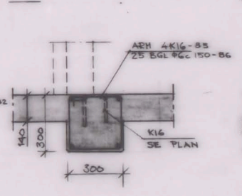
PELARE 405 G 1:10
