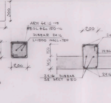
PELARE 504 G 1:10
