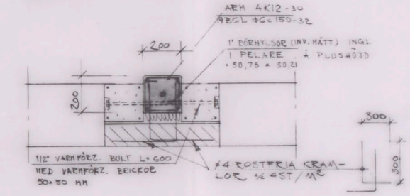
PELARE 504 G 1:10
