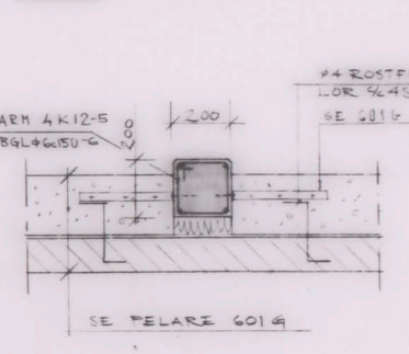
PELARE 605 G 1:10
