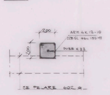
PELARE 604 G 1:10
