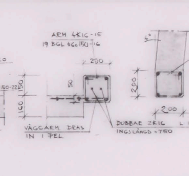
PELARE 505 G 1:10
