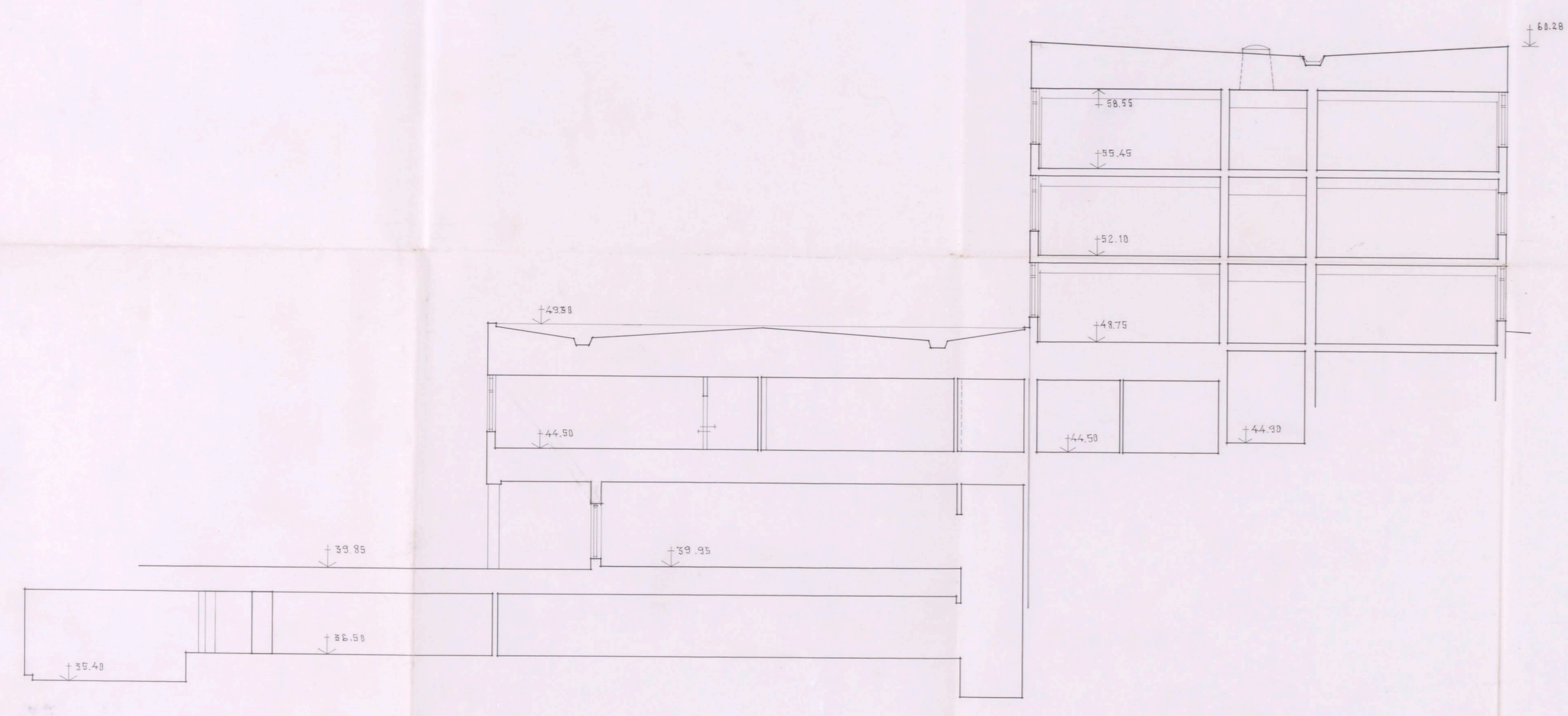
SEKTION A4-A4
