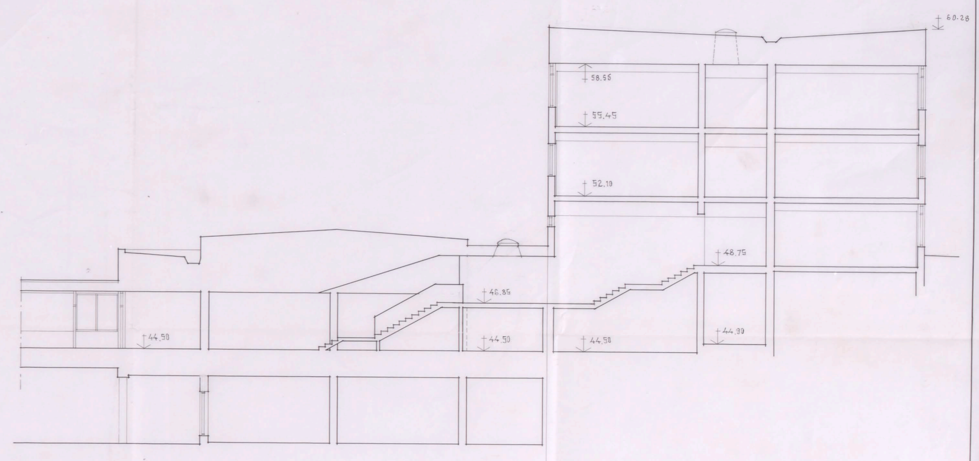
SEKTION A5-A5
