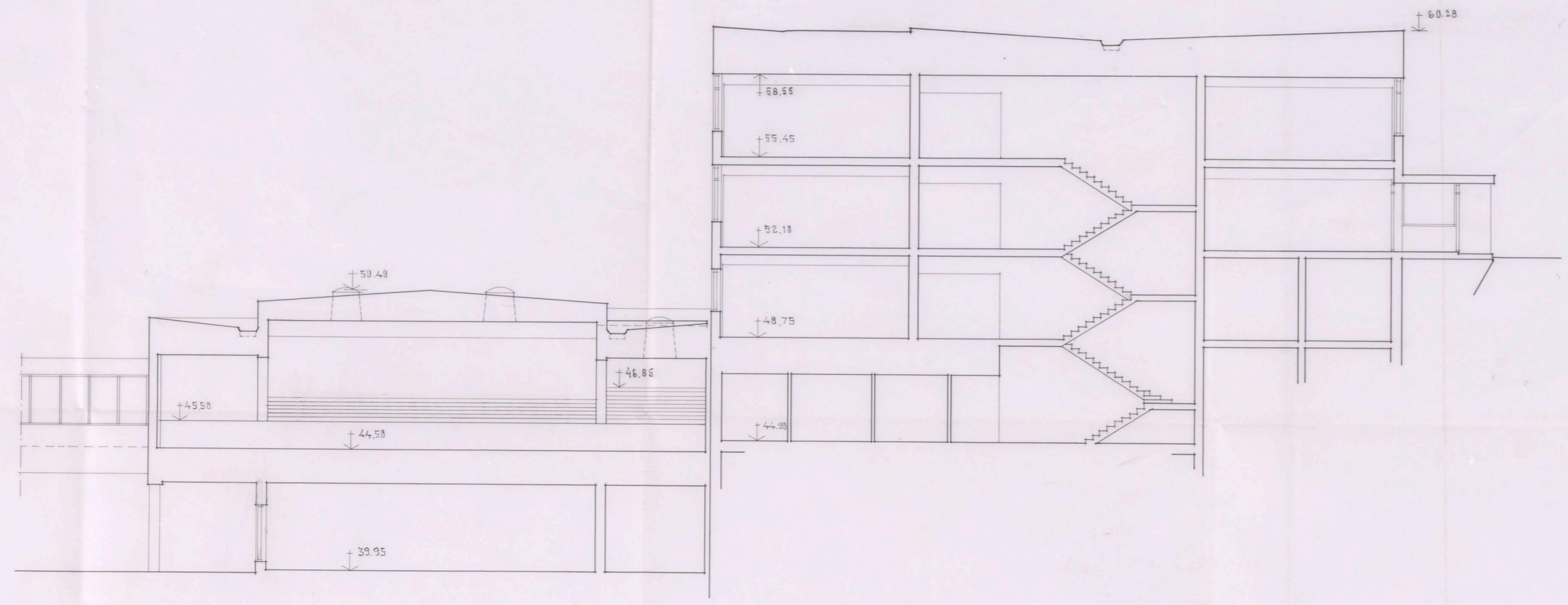
SEKTION A2-A2
