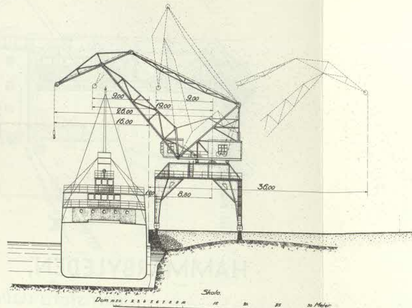
SÖDRA HAMMARBYHAMNEN. SEKTION GENOM ALLMÄNNA LOSSNINGSPLOTSSEN.
