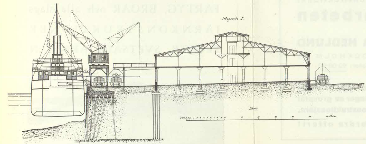
FRIHAMNEN. SEKTION GENOM MAGASIN I.
