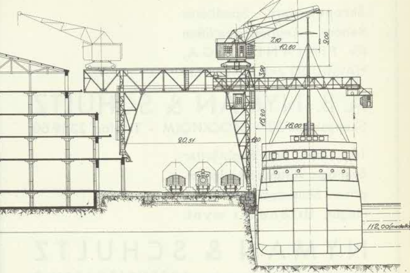
FRIHAMNEN. TVÄRSEKTION GENOM PIREN OCH SÖDRA BASSÄNGSKAJEN.
