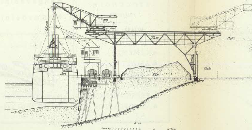
VÄRTAHAMNEN. SEKTION GENOM SÖDRA KAJEN MED MALMKRAN. Kranens lyftförmåga = 10 ton.
