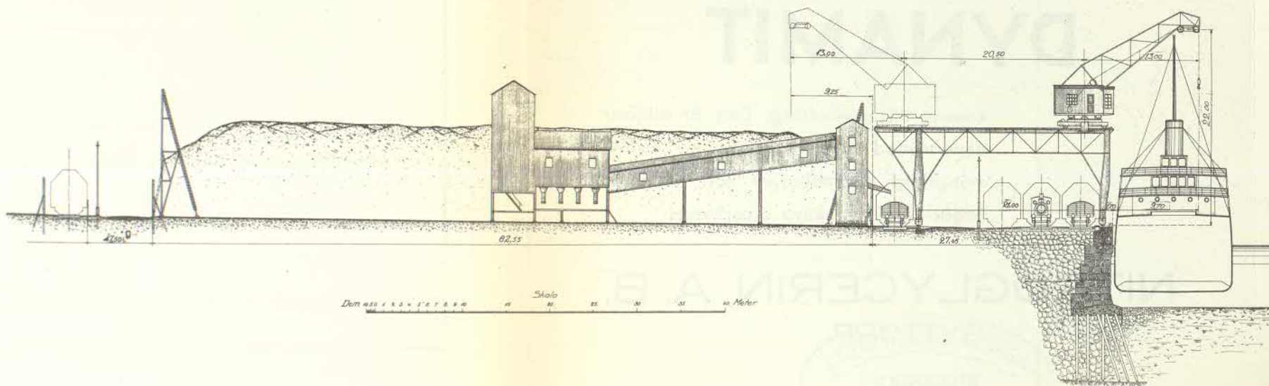
NORRA HAMMARBYHAMNEN. TVÄRSEKTION GENOM BLECKTORNSKAJEN.
