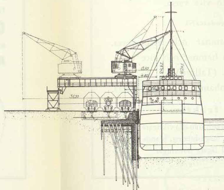
FRIHAMNEN. SEKTION GENOM YTTRE DELEN AV PIREN.
