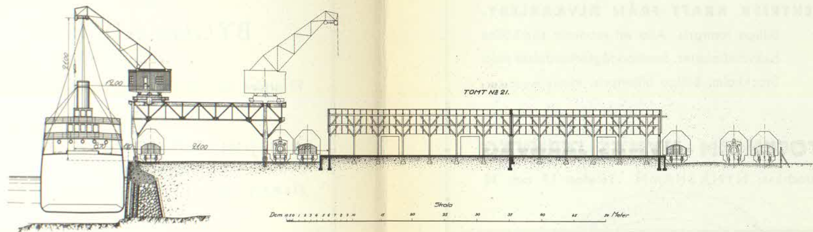
VÄRTAHAMNEN. SEKTION AV SÖDRA BASSÄNGSKAJEN VID TOMT N:O 21.
