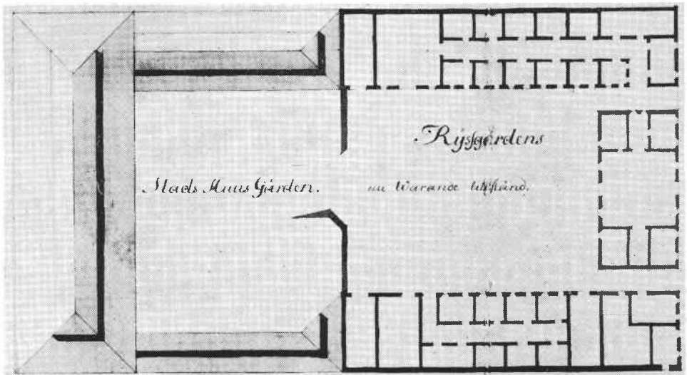
Bild 4. Den på 1690-talet i tegel och korsvirke nyuppförda Ryssgården. Uppmättningsritning av stadsarkitekten J.E. Carlberg 1743. »Den war af 77 alnars längd på båda sidor och bredd 84 alnar, omgifwen med 29 st. bodar och Magazin». — Mellan flyglarna våghuset med 4 st. kontor. I södra flygeln, ovanpå bodarna, var Ryska kyrkan. Magasinen skiljas från de mot gården vettande bodarna av en korridor. — (Stadsarkivets ritningssamling 144: 20.)
