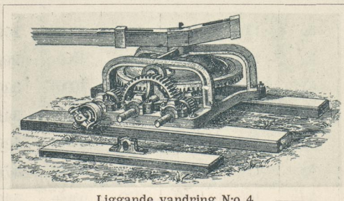
Liggande vandring No 4 för 1 å 2 dragare. Vigt: 360 kg. Pris: Kr. 175.—
