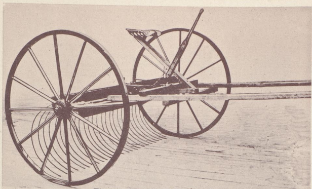
Tigerräfsa, sjelfafläggande
