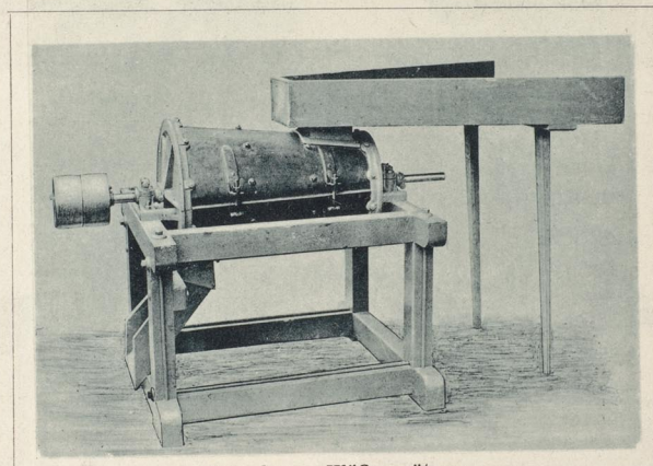
Israelssons Klöfvernötare
