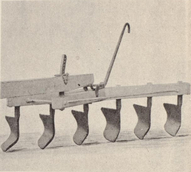
Myllharf med vändskifvor
