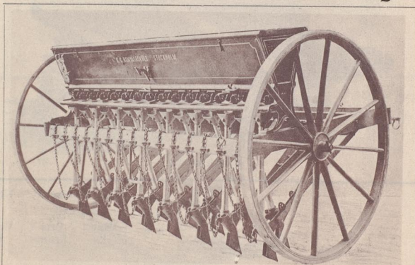
Champion-radsåningsmaskin
