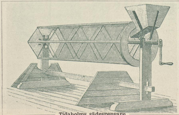
Tidaholms sädesrensare
