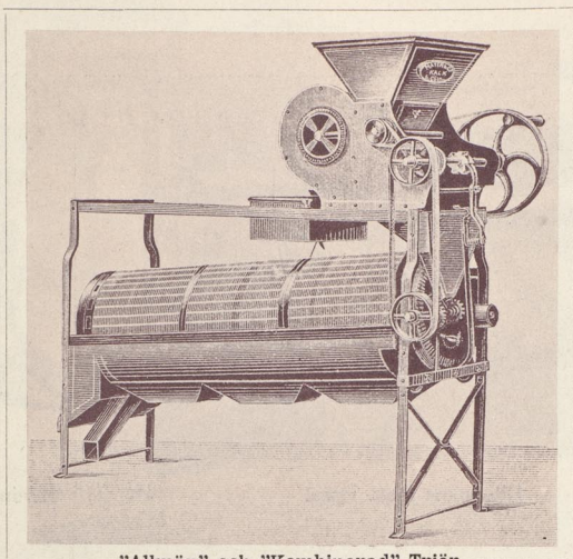
"Allmän" och "Kombinerad" Triör med skaksäll och fläkt
