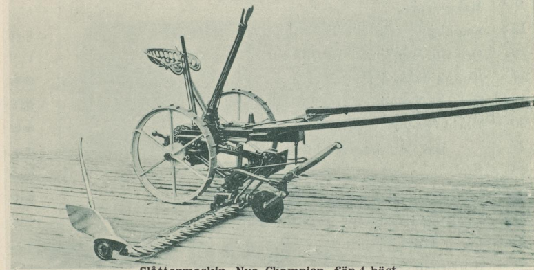
Slättermaskin, Nya Champion, för 1 häst
