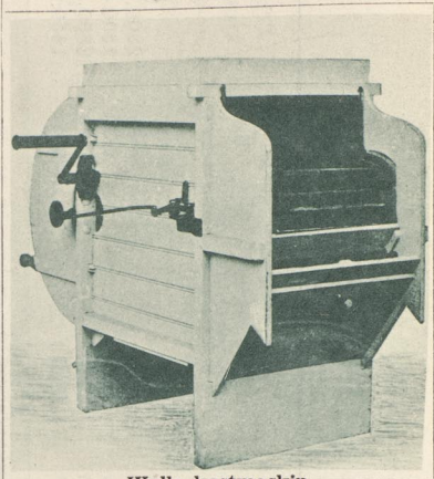
Walla kastmaskin
