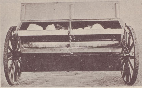
Gödselspridningsmaskin Svea Vigt: 160 kg. Pris: Kr 225.—
