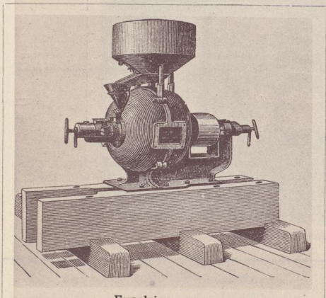
Excelsior-quvarn med franska stenar
