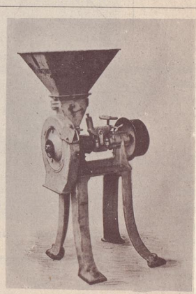
Excelsior-quvarn med stålskifvor
