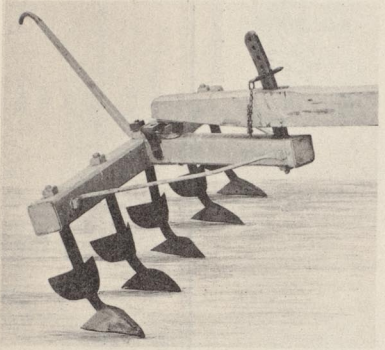
Myllharf med billar
