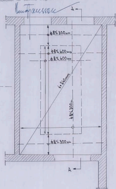
Bjälklag över vänstra trappan
