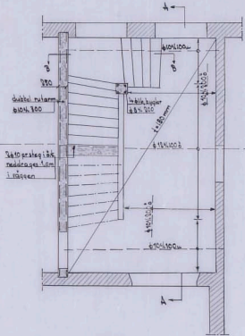
Bjälklag över våning 1 trappa
