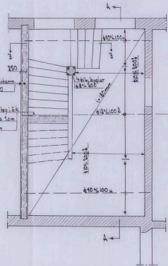
Bjälklag över bottenvåning
