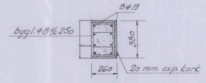
Sektion F9-F9
