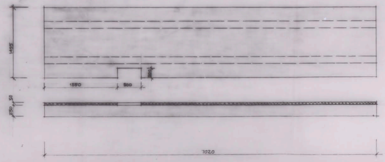
KASSETT 5 V ANTAL 1 ST 1:20
