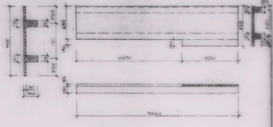
KASSETT 18 V ANTAL 1 ST 1:20
