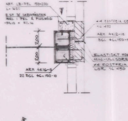
DETALJ 715 G 1:10 GM BRÖSTNING SE DET 707 G
