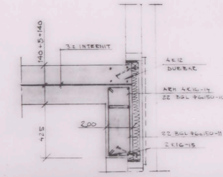
DETALJ 712 G 1:10 GÄLLER BILG 400 BILG 300 I PRINCIP
