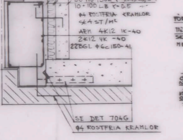
DETALJ 714 G 1:10 BILG 500
