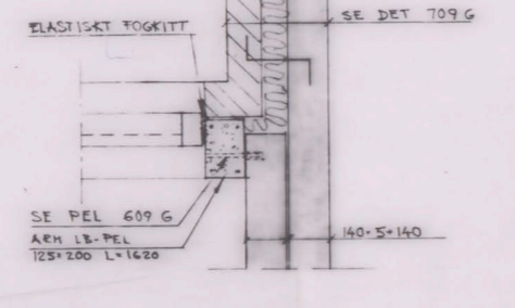
DETALJ 710 G 1:10 BILG 600
