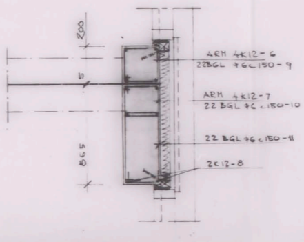
DETALJ 712 G 1:10 GENOM BRÖSTNING GÄLLER ÄVEN BILG 600 I PRINCIP
