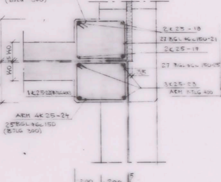
DETALJ 712 G 1:10 BILG 200
