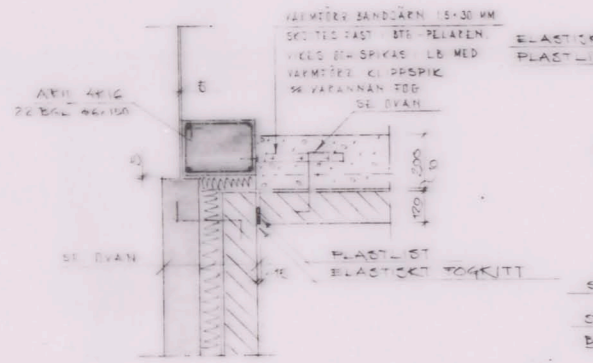
DETALJ 700 G 1:10 GÄLLER BILG 400
