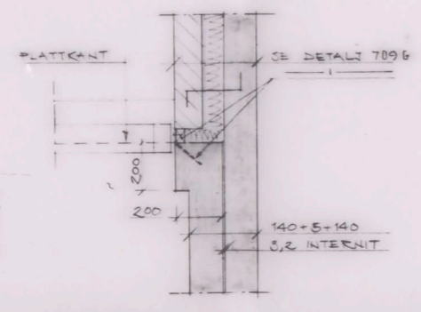
DETALJ 710 G 1:10 GENOM BRÖSTNING GÄLLER ÄVEN BILG 600
