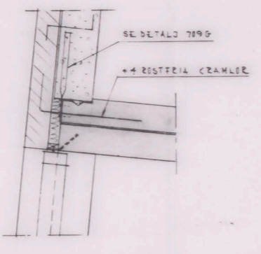
DETALJ 711 G 1:10 GÄLLER BILG 400 & 300
