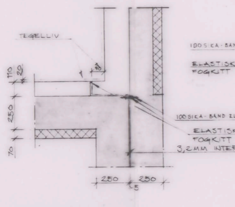
DETALJ 710 G 1:10 BILG 600
