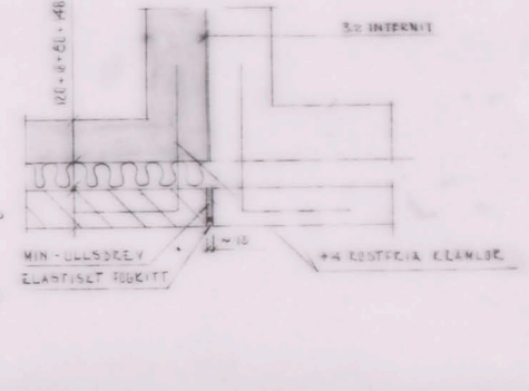
DETALJ 713 G 1:10 BILG 300
