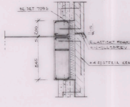
DETALJ 712 G 1:10 BILG 600
