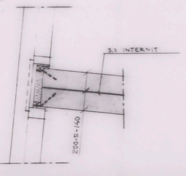
DETALJ 711 G 1:10 GENOM BRÖSTNING GÄLLER ÄVEN BILG 500 & 600
