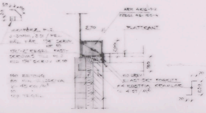
DETALJ 700 G 1:10 GENOM BRÖSTNING GÄLLER ÄVEN BILG 600 & 500
