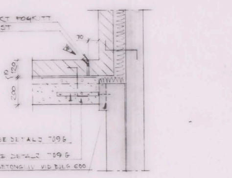
DETALJ 710 G 1:10 GÄLLER BILG 500 400 I PRINCIP
