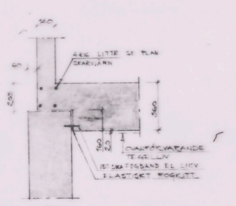
DETALJ 709 G 1:10 GÄLLER BILG 500
