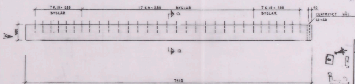
BALK B C10 H ANTAL - 1 ST 1:20
