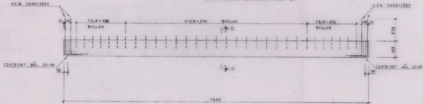
BALK B C03 H ANTAL - 1 ST, B C08 H ANTAL - 15 ST, B C02 G ANTAL - 25 ST 1:20
