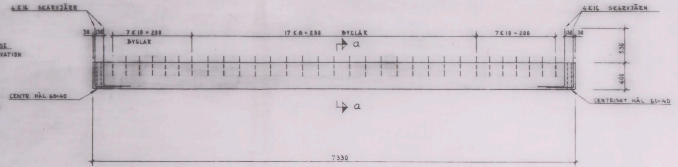
BALK B C04 H ANTAL - 9 ST 1:20
