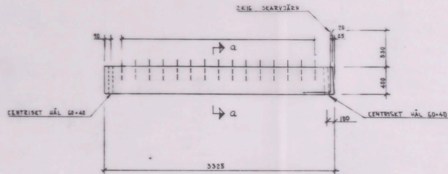
BALK B C10 H ANTAL - 1 ST 1:20
