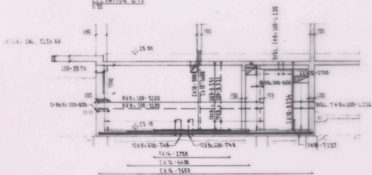
ELEVATION B 13 1:50
