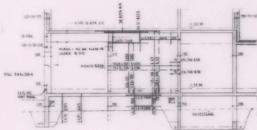
ELEVATION A 13 1:50
