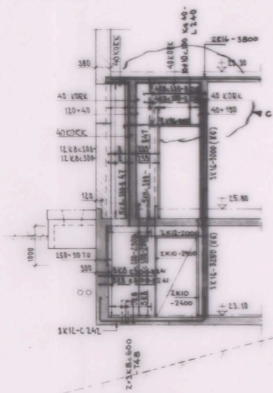
ELEVATION D 13 1:50
