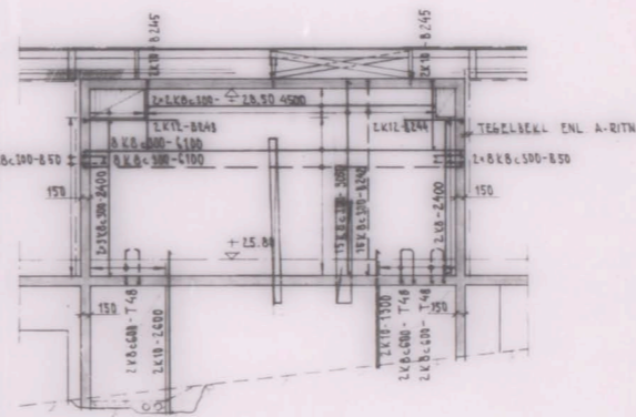
ELEVATION E 13 1:50
