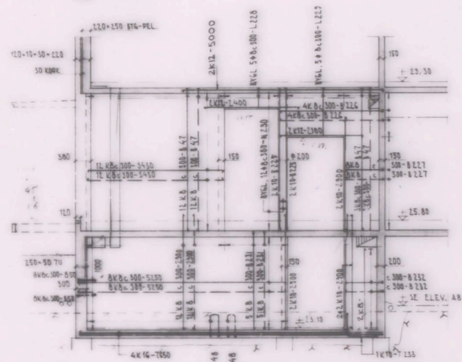
ELEVATION A 13 1:50
